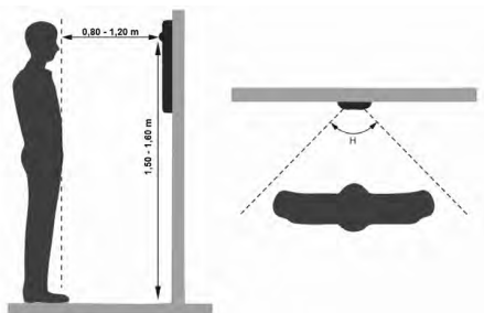
Abbildung 3-1 Installationsort-Referenz
