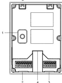
Abbildung 2-2 Geräterückseite
