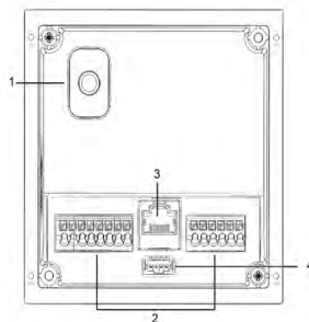
Abbildung 2-2 Kameramodul (Rückseite)
