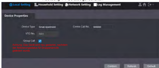
Abbildung 4-4 Geräteeigenschaften
