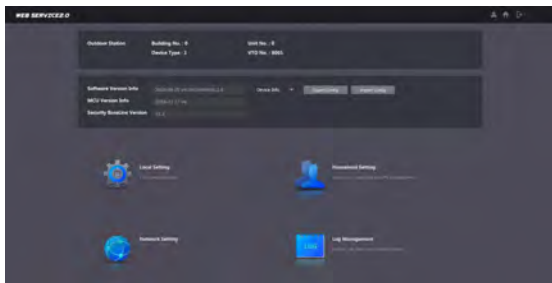
Abbildung 4-3 Hauptfenster
