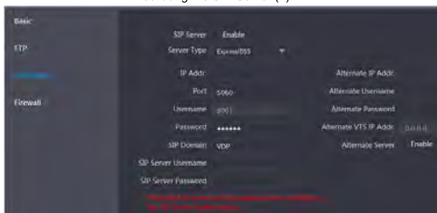
Abbildung 4-8 SIP-Server (2)
